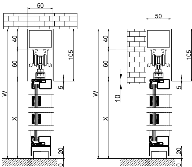
Deckenmontage
